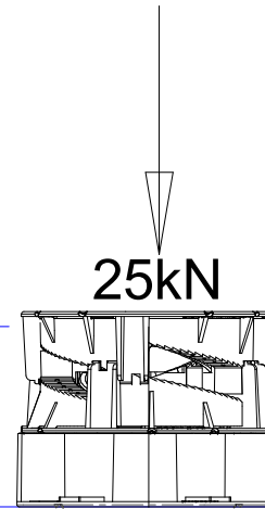
SP-T44+45E 105-119mm
